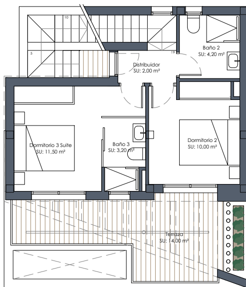
Planta Primera
