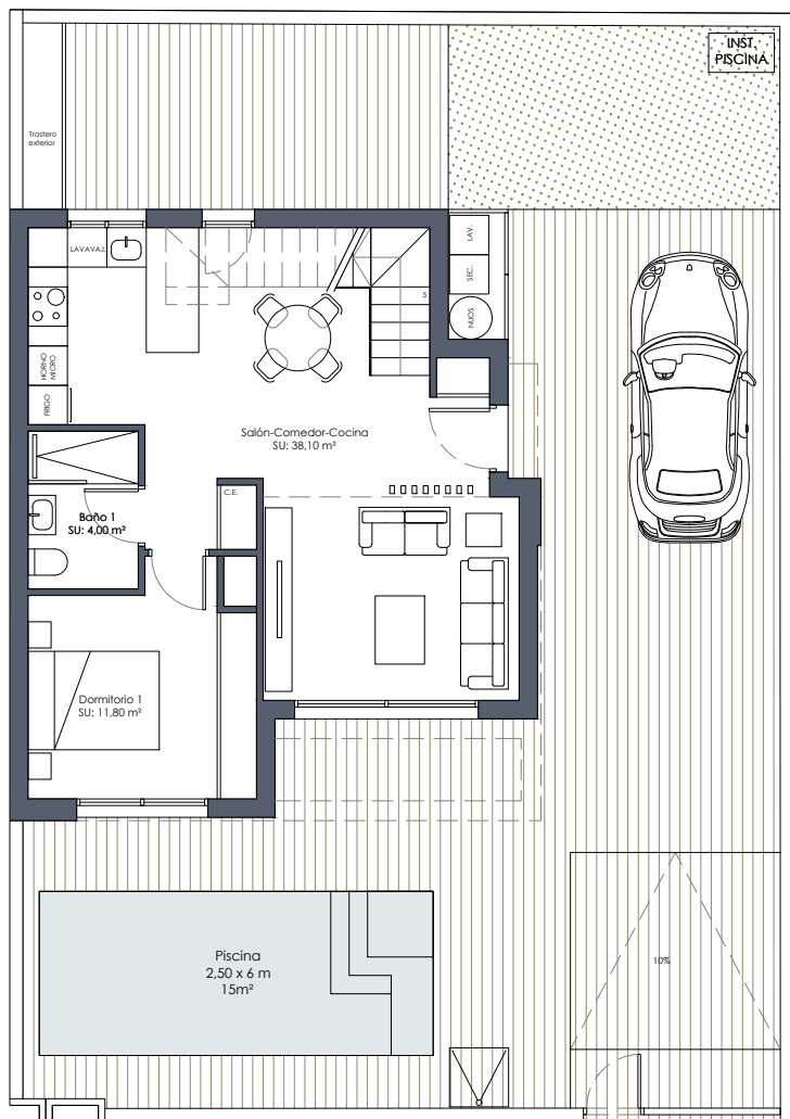
Planta Baja
