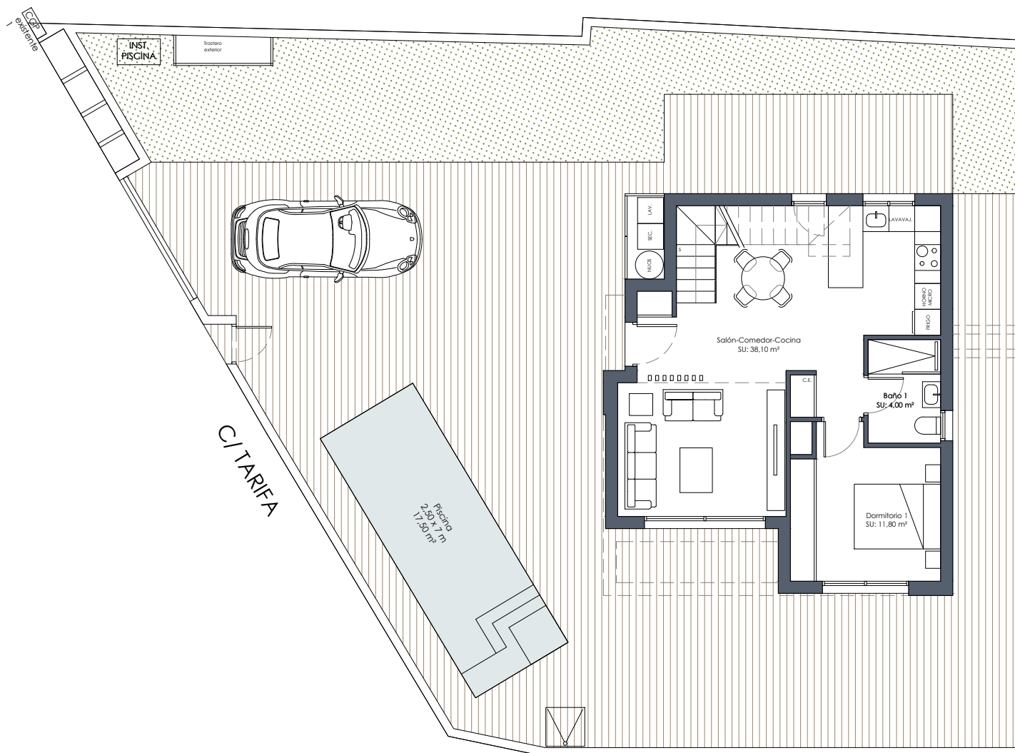
Planta Baja
